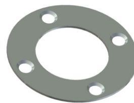
DISCO DE ENCOSTO 3LE 32541 BALANÇA CÓD.: 30024
