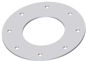
JUNTA DO TAMBOR DE SECAGEM DO FELTRO DES. 60-2157 CÓD.: 116424
