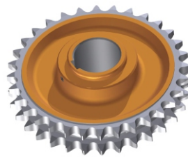
ENGRENAGEM DUPLA Z32 DES. 55-1518 CÓD.: 105352
